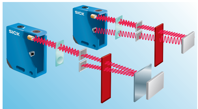
▼ Polarisation filter
