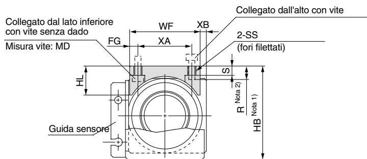
Viste D-D'
