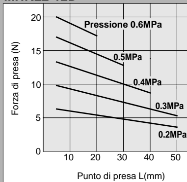
MHKL2-16D
