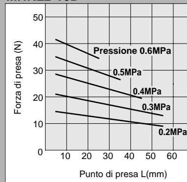
MHKL2-20D
