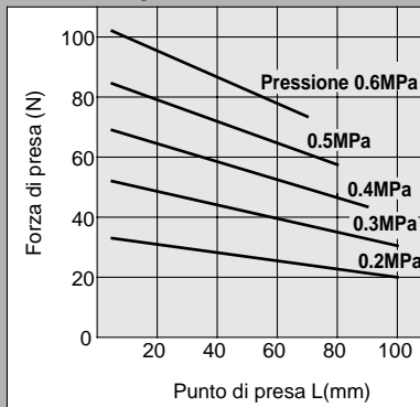
MHKL2-25D
