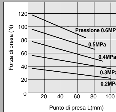
MHKL2-25D
