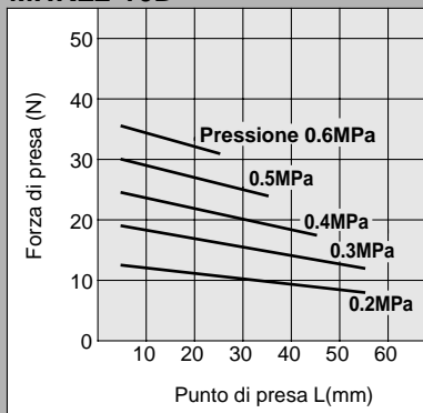
MHKL2-20D
