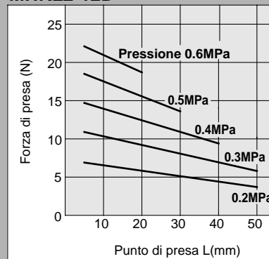
MHKL2-16D
