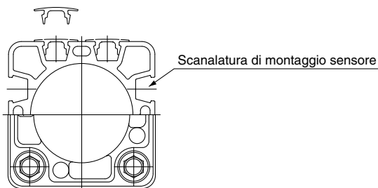
Vista trasversale
