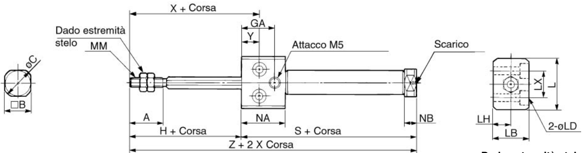
Dado estremità stelo
