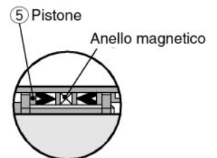
Costruzione del pistone in caso di dotazione sensori
