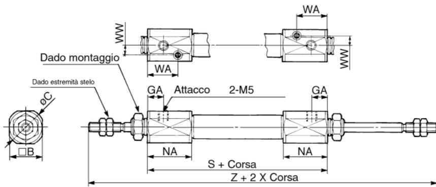
Dado estremità stelo
