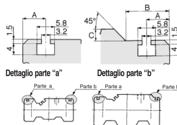
MGQ□32 ÷ 50 MGQ□63 ÷ 100
