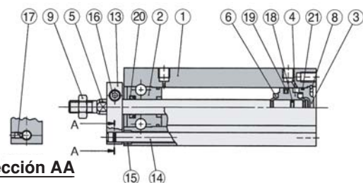
Sección AA
