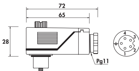
Connettore 2
